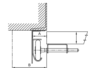
STEEL JAMB
