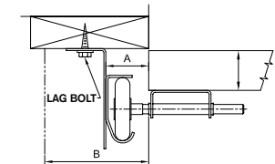
WOOD JAMB
